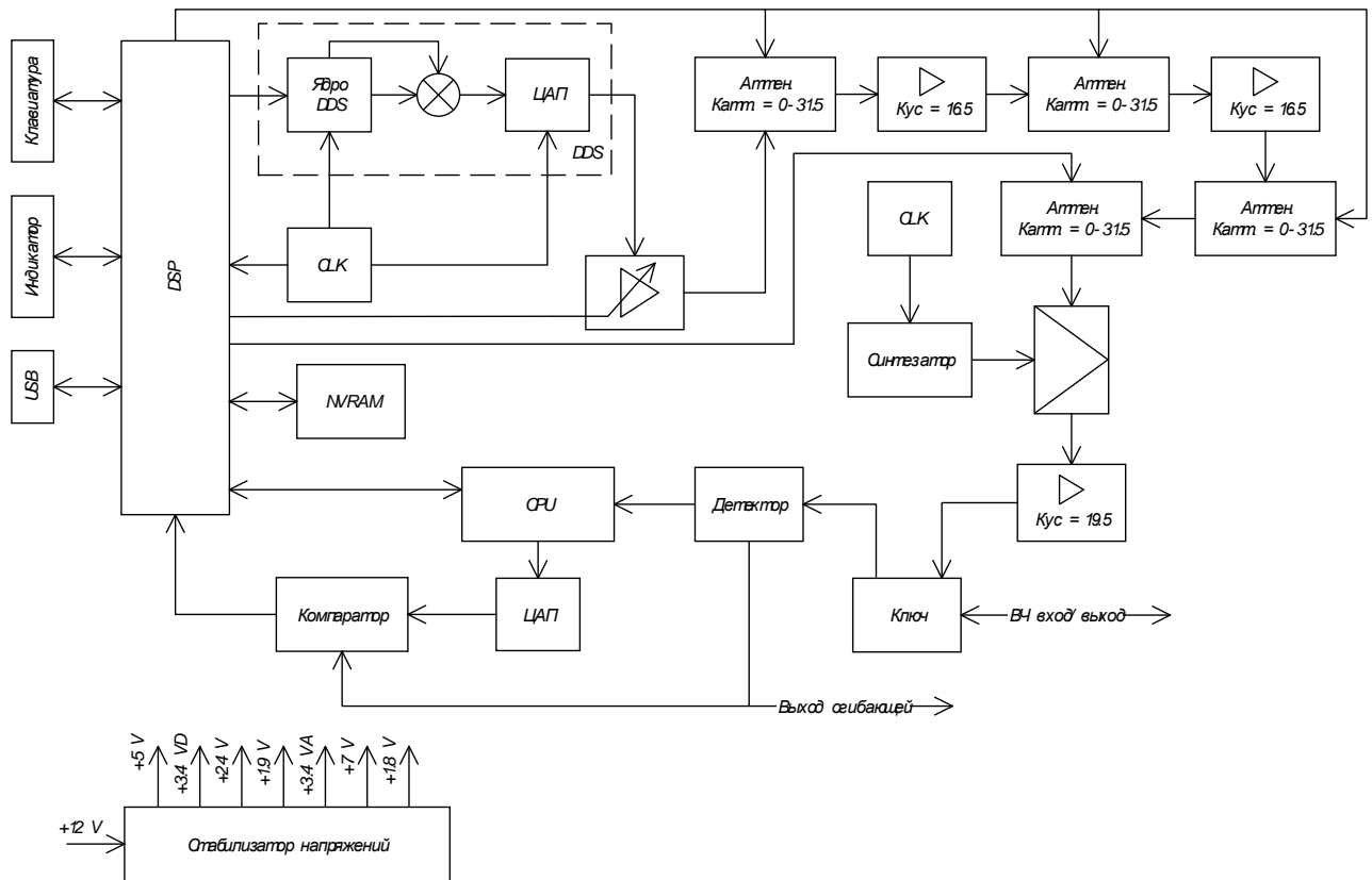
Рис.1. Функциональная схема
